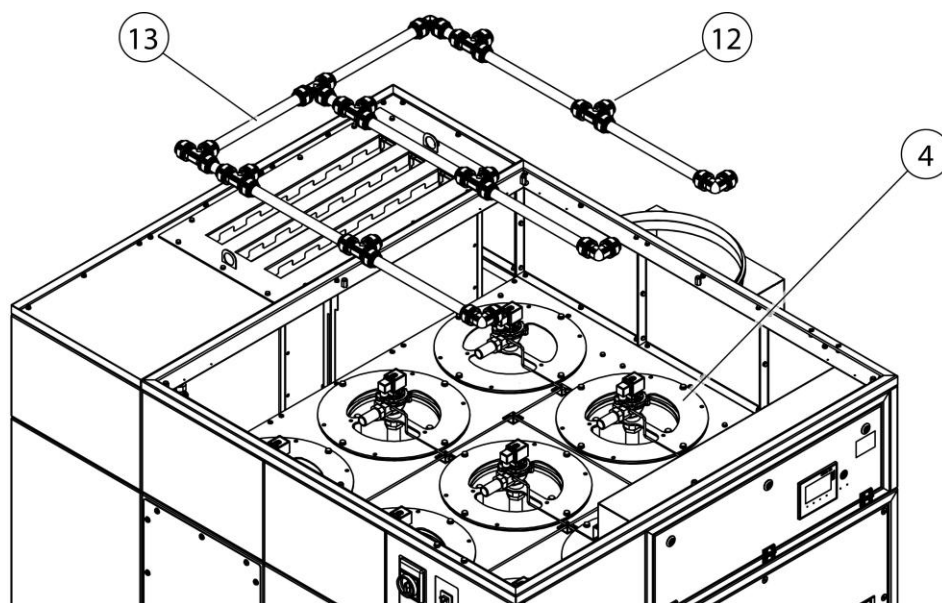
Fig. 44: Filterbytte – demontere trykklufttrør
