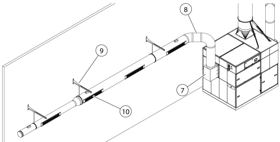
Fig. 14: Veggmontering - inntaksrør
