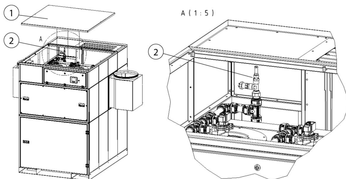
Fig. 53: tilgang til trykkluft-sikkerhetsventilen
