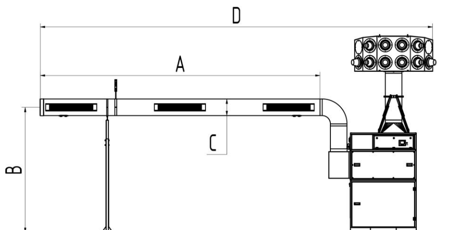
Fig. 57: Målskisse – 998800407
