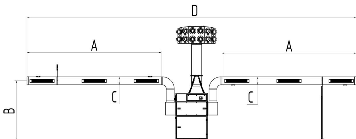
Fig. 58: Målskisse – 998800401
