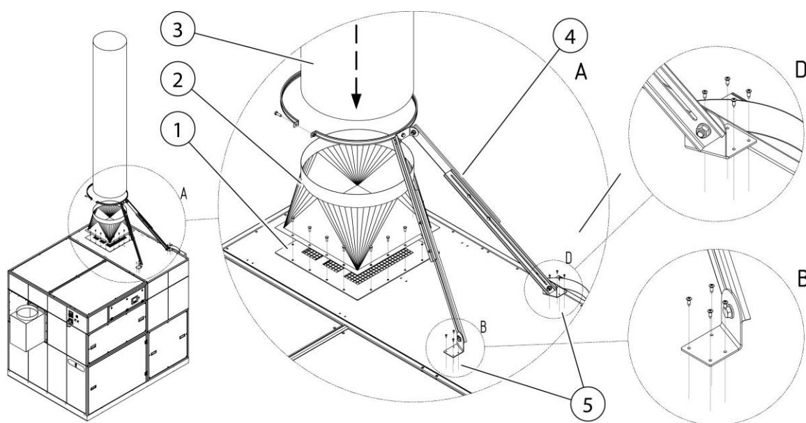
Fig. 12: Montering - utblåsningsenhet
