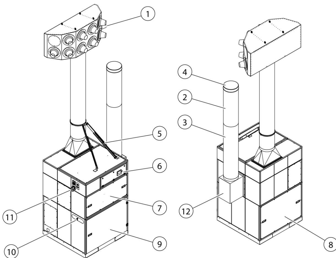
Fig. 4: Funksjonsbeskrivelse - 998800461
