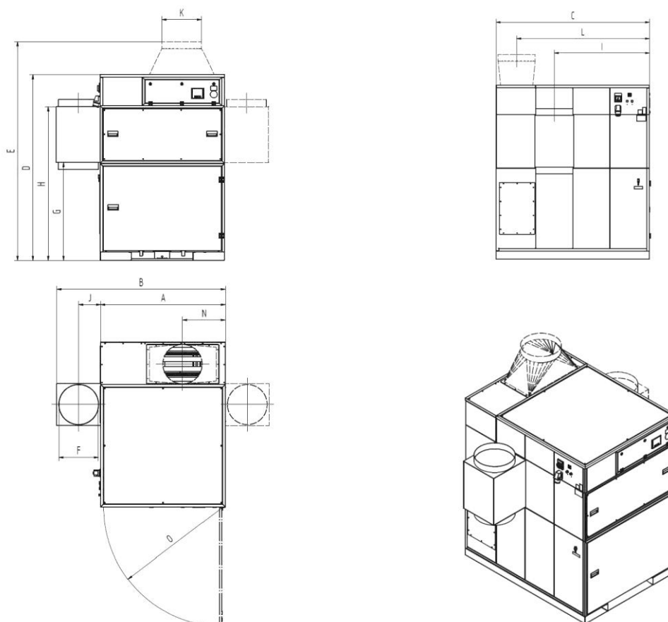
Fig. 55: Måleskisse 998701371 (998800401, 998800462)
