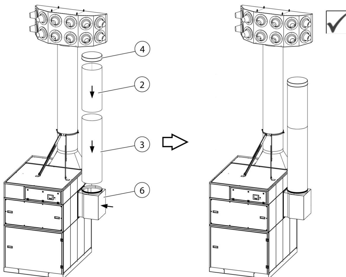
Fig. 17: Posisjoner på produktet
