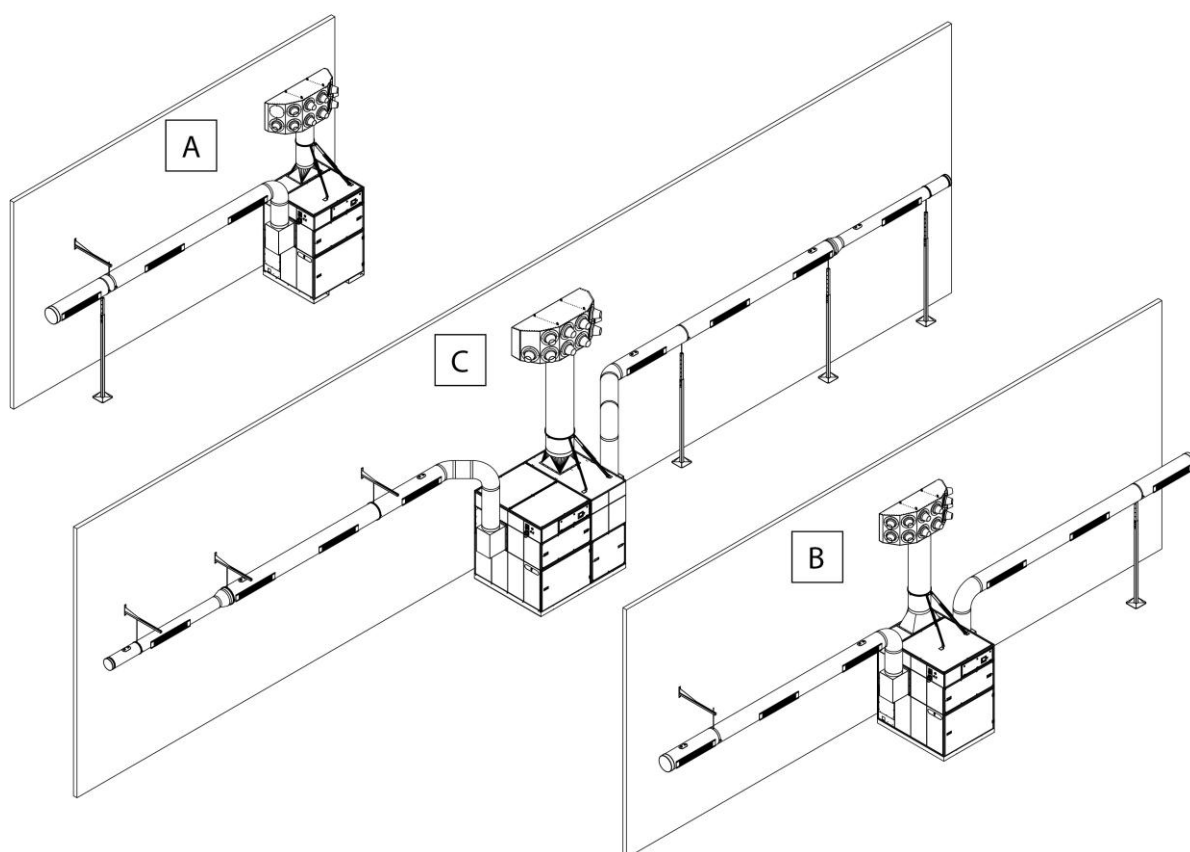
Fig. 11: Montering – oversikt over produktvariantene
