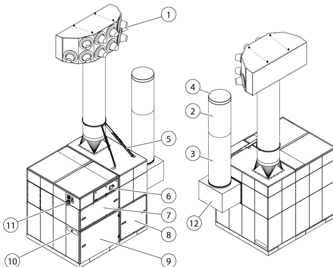
Fig. 6: Funksjonsbeskrivelse - 998800463
