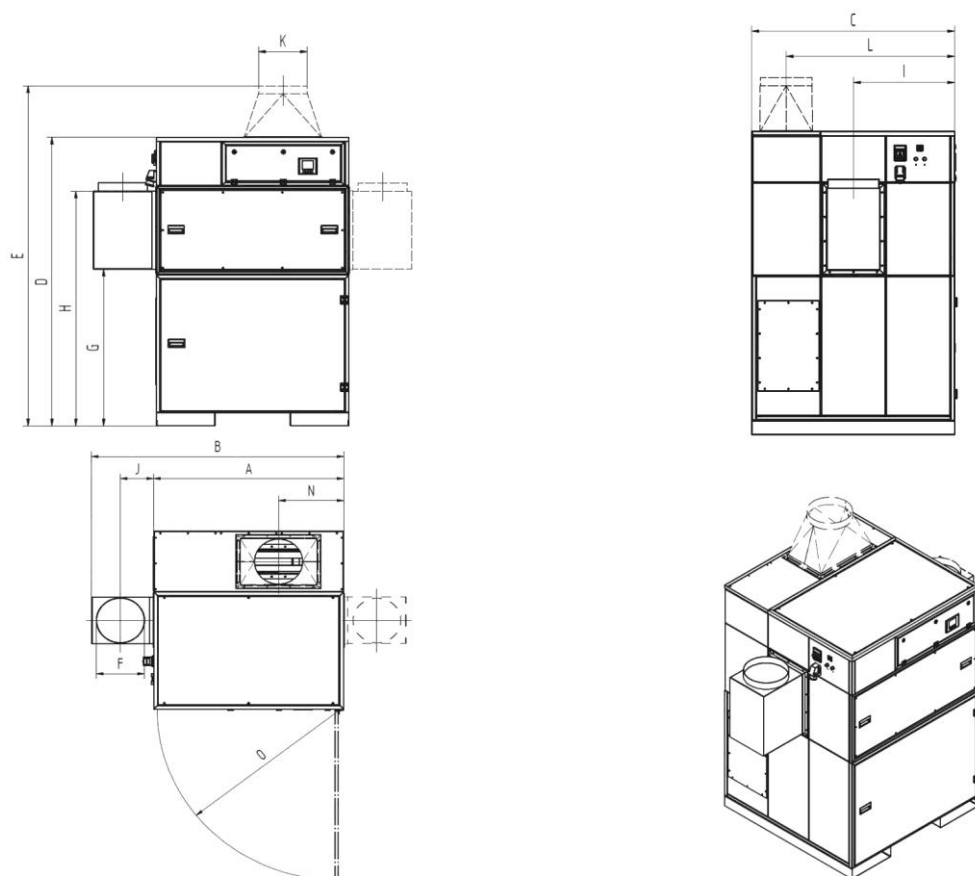
Fig. 54: Måleskisse 998701372 (998800407, 998800461)
