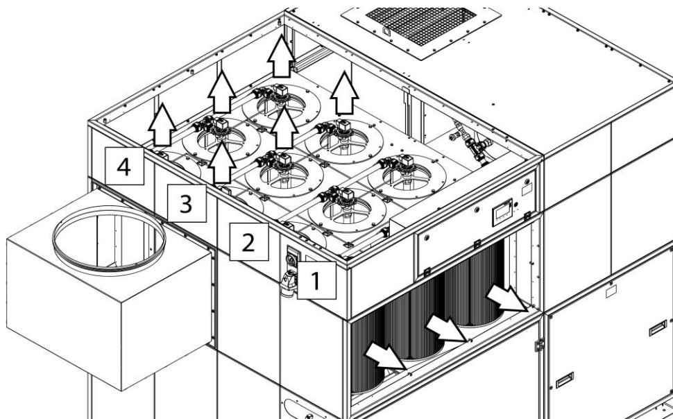
Fig. 39: Filterbytte
